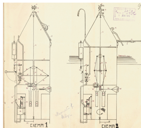
Материалы об испытании аппарата для выпуска почтовых голубей из погруженной подводной лодки. Схема. 1929 г. РГАВМФ
